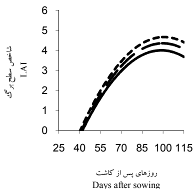
شکل ۴- شاخص سطح برگ ذرت در تراکم ۹/۵۲ بوته در متر مربع Fig. 4. Leaf area index of maize in 9.52 plant.m -2 density Single تک ردیفه (—): Y = -0.001x^2 + 0.244x - 8.096 ; R^2 = 0.85 Twin دو ردیفه (---): Y = -0.001x^2 + 0.253x - 8.293 ; R^2 = 0.84 Zigzag زیگزاگ (....): Y = -0.001x^2 + 0.257x - 8.324 ; R^2 = 0.85
