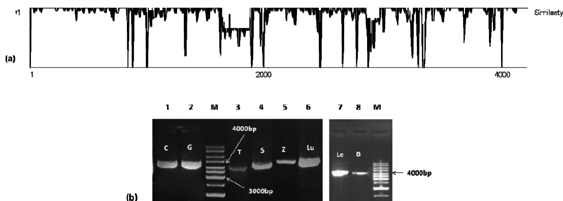
شکل ۱- (a) آنالیز شباهت ناحیه هدف گیری کننده به ژنوم کلروپلاستی جداشده از ژنوم‌های پلاستییدی هویج، کاهو، پنبه،
