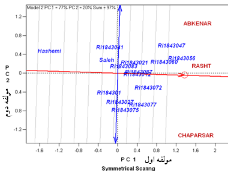
شکل ۲ - نمودار دو بعدی مختصات تستر متوسط بای پلات برای بررسی همزمان پایداری و عملکرد ژنوتیپ‌های برنج Fig. 2. Average tester coordination (ATC) views of the GGE-biplot for performance and stability of the rice genotypes
