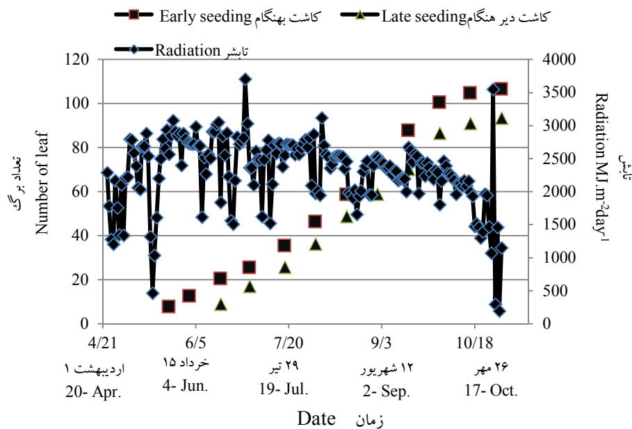
شکل ۳- روند تولید برگ چغندر قند و تابش خورشید در دو زمان کاشت (۱۳۹۰ و ۱۳۸۹)
