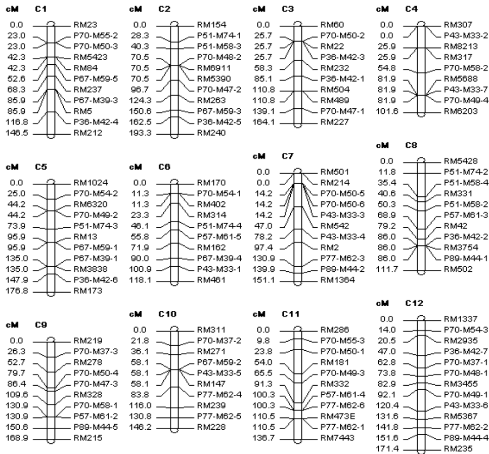
شکل ۲- نقشه پیوستگی ۱۲۸ نشانگر SSR و AFLP در جمعیت F 2 حاصل از تلاقی ارقام برنج بینام و کادوس. نشانگرها در سمت راست گروه‌های پیوستگی و فاصله ژنتیکی آن‌ها بر اساس تابع کوسامبی در سمت چپ آن‌ها نشان داده شده است. گروه‌های پیوستگی بر
