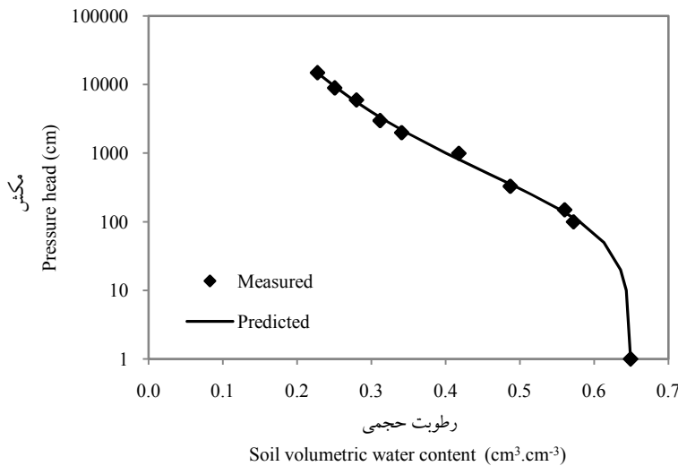
شکل ۱- منحنی مشخصه رطوبتی در خاک مورد مطالعه Fig. 1. Characteristic moisture curve of studied soil
