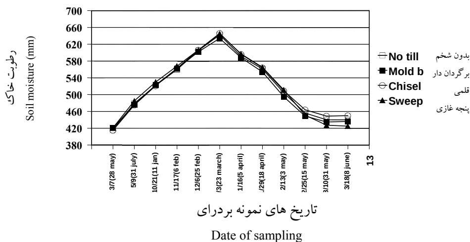
شکل ۴- اثر ادوات شخم بر رطوبت خاک تا عمق ۱۸۰ سانتیمتر در سال زراعی ۱۳۶۶-۶۷
