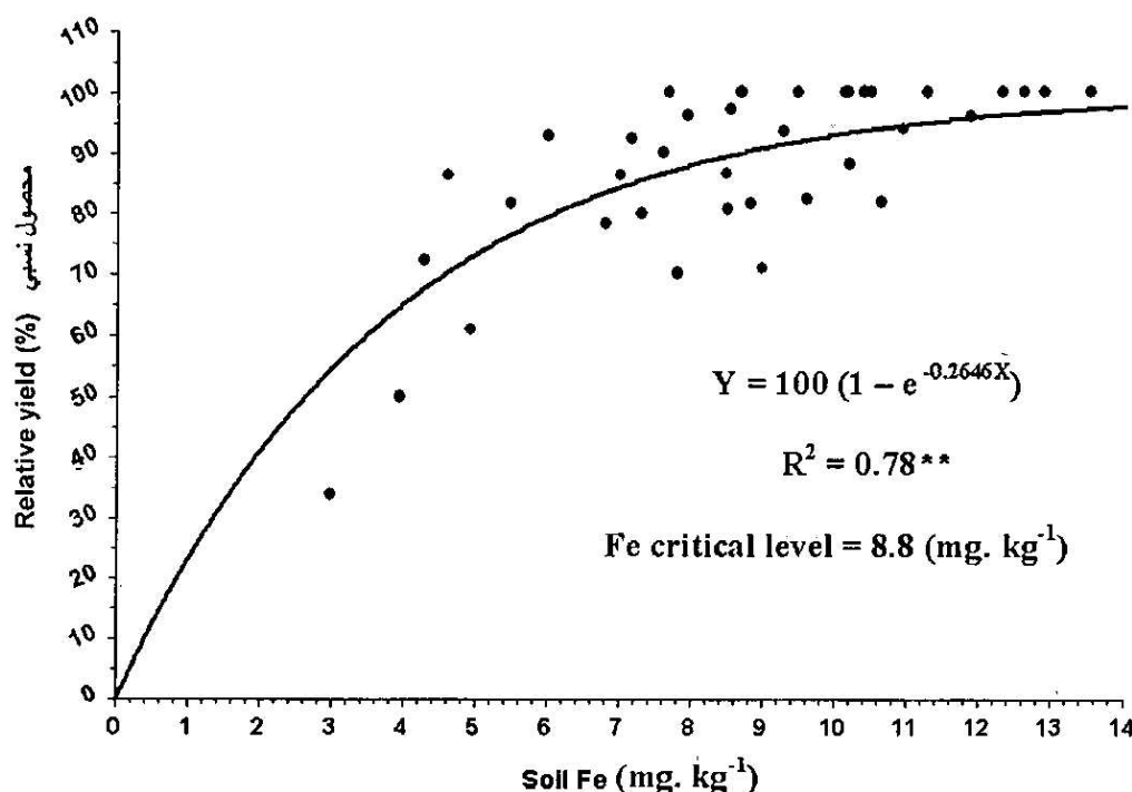
شکل ۱- حد بحرانی آهن در خاک برای گندم دیم در شمال غرب کشور با استفاده از معادله میچرلیش Fig. 1. Soil Fe critical level for dryland wheat in the northwest of Iran using Mithscherlich equation
