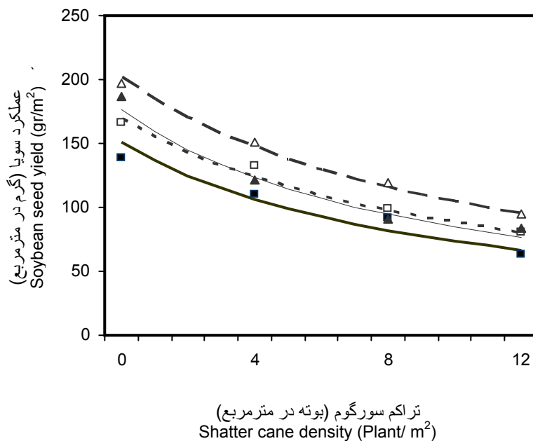
شکل ۲- روند تغییرات عملکرد سویا در واحد سطح و تراکم سورگوم در تراکمهای ۲۰ (■——■)، ۳۰ (□-----□)، ۴۰ (Δ——Δ) و ۵۰ (▲-----▲) بوته در مترمربع سویا
