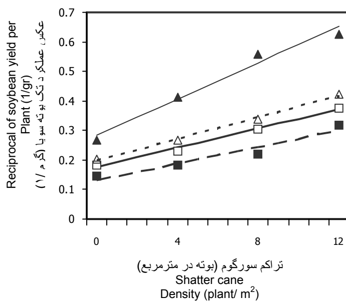
شکل ۱- روند تغییرات عکس عملکرد تک بوته سویا ۲۰ (■-----■)، ۳۰ (□——□)، ۴۰ (Δ-----Δ) و ۵۰ (▲——▲) تراکم سورگوم در تراکمهای ۲۰، ۳۰، ۴۰ و ۵۰ بوته در مترمربع سویا
