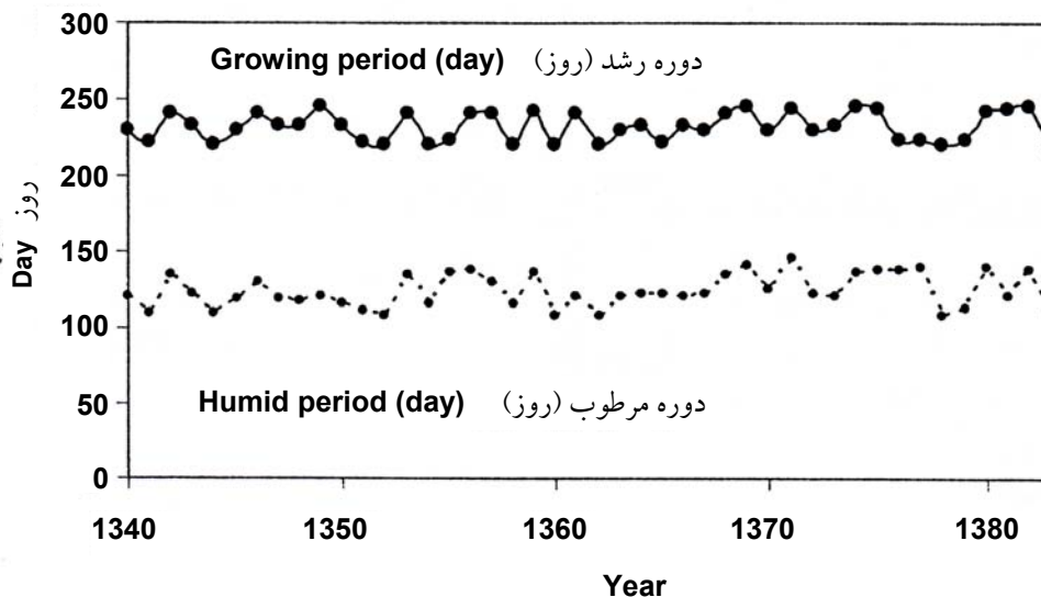
شکل ۴- تغییرات زمانی طول دوره رشد و طول دوره مرطوب از سال ۱۳۴۰ تا سال ۱۳۸۳ در منطقه مورد مطالعه Fig. 4. Temporal variability of length of growing and humid periods in the study area for 1961-2004
