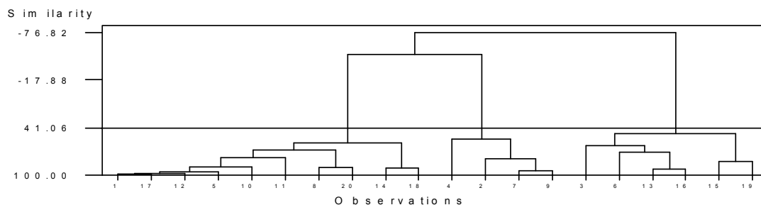
۱- دندوگرام حاصل از تجزیه خوشه ای \alpha ذرت بر اساس شاخص های تحمل و حساسیت به تنش و عملکرد دانه
