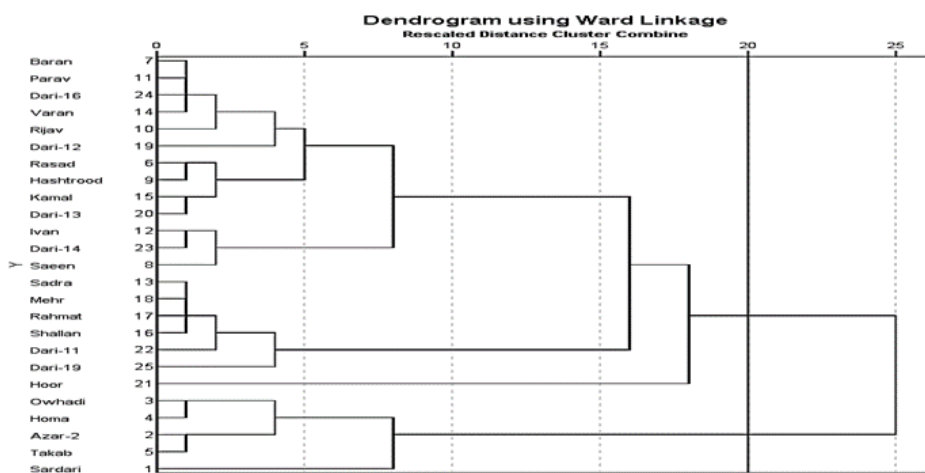
شکل ۱- دندروگرام حاصل از تجزیه خوشه‌ای برای صفات و شاخص‌های گیاهی ارقام گندم در تیمار آبیاری کامل (بدون تنش) Fig. 1. Dendrogram of cluster analysis for plant traits and indices of wheat cultivars in full irrigation (normal) treatment
