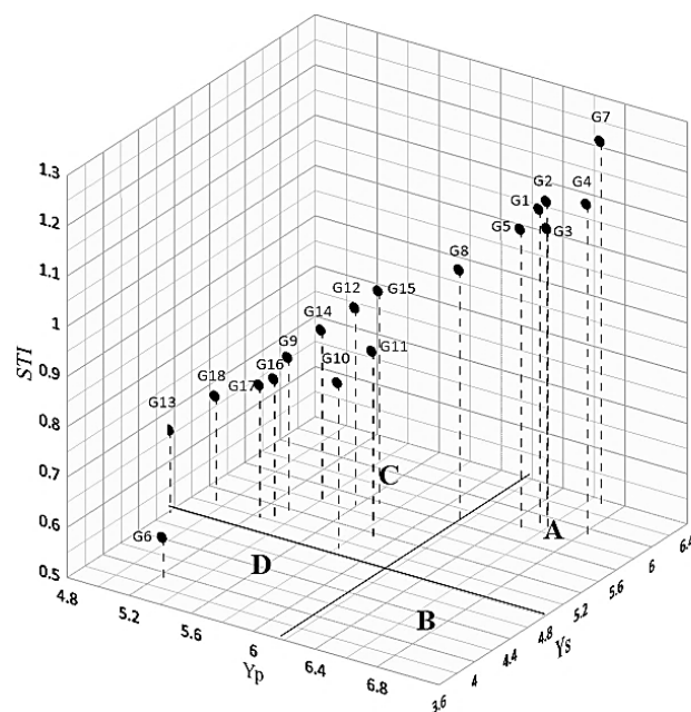
شکل ۳- نمودار سه بعدی عملکرد دانه ژنوتیپ‌های جو در شرایط بدون تنش (Yp)، تنش خشکی انتهایی فصل (Ys) و شاخص STI (۱۴۰۲-۱۴۰۳ و ۱۴۰۱-۱۴۰۲)
