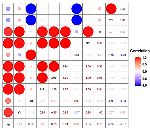
شکل ۲- ضرایب همبستگی بین عملکرد دانه ژنوتیپ‌های جو و شاخص‌های ارزیابی تنش در شرایط بدون تنش (Yp) و تنش خشکی انتهایی فصل (Ys)
