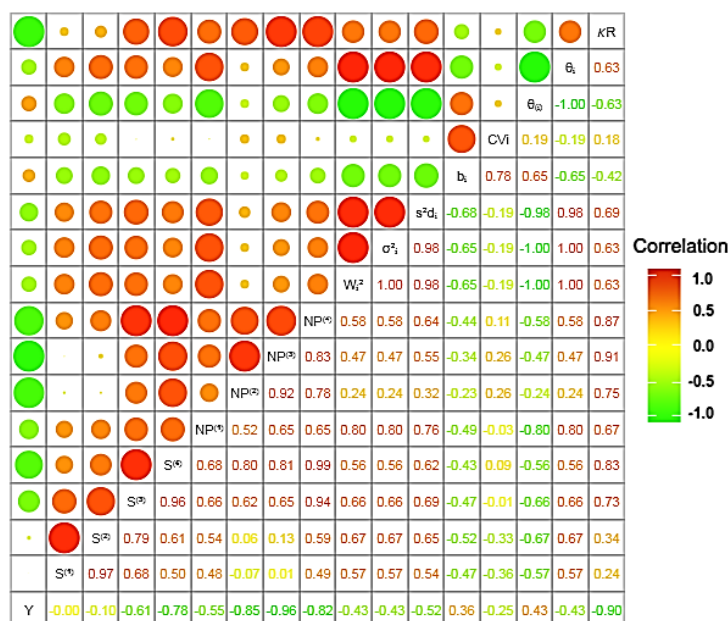
شکل ۱- ضرایب همبستگی بین عملکرد دانه و آماره‌های پارامتری و ناپارامتری پایداری در ژنوتیپ‌های جو
