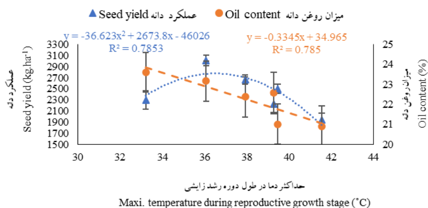
شکل ۸- رابطه رگرسیونی بین عملکرد دانه و میزان روغن دانه با حداکثر دما در طول دوره رشد زایشی ژنوتیپ‌های سویا Fig. 8. Regression relationship between seed yield and seed oil content with maximum temperature during reproductive stage of soybean genotypes
