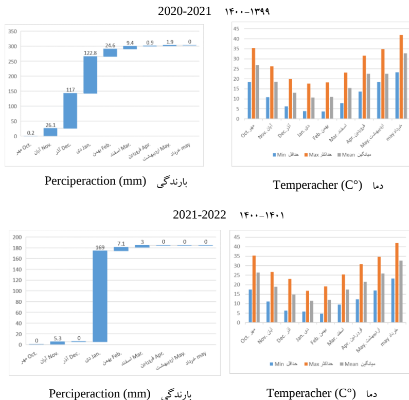
شکل ۱- اطلاعات هواشناسی محل اجرای آزمایش (۱۳۹۹-۱۴۰۰ و ۱۴۰۰-۰۱)
