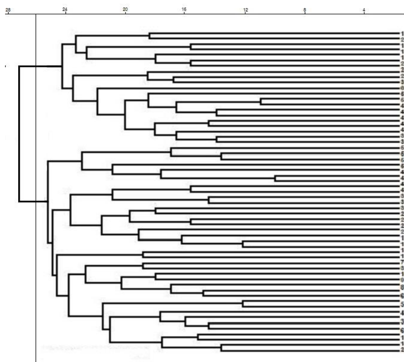
شکل ۲- دندروگرام تجزیه خوشه‌ای برای گروه بندی ۶۰ ژنوتیپ کینوا با استفاده از ۴۰ نشانگر ریزماهواره
