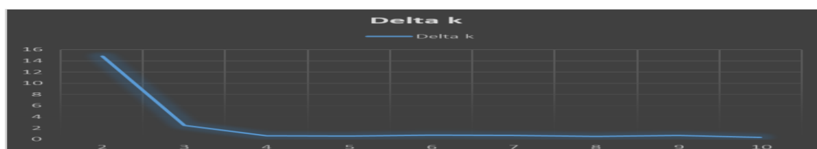
شکل ۳- نمودار دوسویه برای شناسایی تعداد مناسب زیرجمعیت در ژنوتیپ‌های کینوا ( K=2 ) با استفاده از نشانگرهای ریزماهواره
