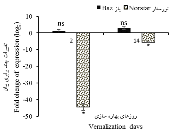
شکل ۴- اثر تیمارهای بهاره‌سازی بر بیان نسبی ژن miR156 در برگ دو رقم گندم باز (بهاره) و نورستار (زمستانه)
