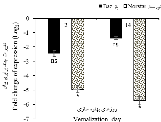
شکل ۵- اثر تیمارهای روزهای بهاره‌سازی بر بیان نسبی ژن SPL3 در برگ دو رقم گندم باز (بهاره) و نورستار (زمستانه)
