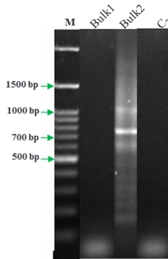
شکل ۱- الگوی نواری بندی بین دو بالک تک شاخه (Bulk1) و چندشاخه (Bulk2) با استفاده از جفت آغازگر MOC1R3/Ga5 کنترل منفی و M نشانگر وزن مولکولی 1Kb است
