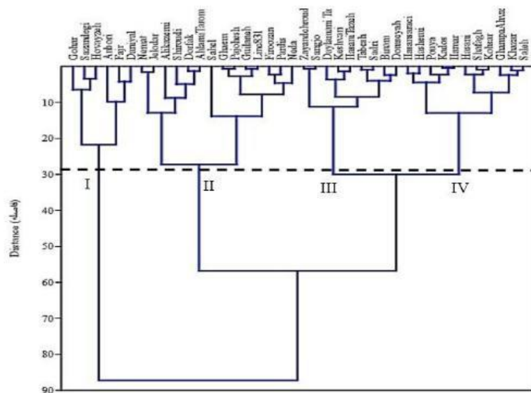
شکل ۱- دندروگرام حاصل از تجزیه خوشه‌ای ژنوتیپ‌های برنج به روش گروه‌بندی واریانس حداقلی (۱۳۹۳) (ضرب کم فنک: ۰/۷۵۱۶)
