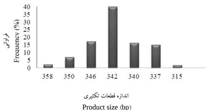
شکل ۲- فراوانی ال‌های تکثیر شده توسط جفت آغازگر Glu3A.2 در ژنوتیپ‌های گندم بومی بهاره ایران
