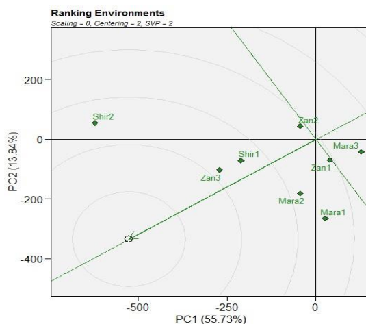
شکل ۶- مقایسه محیط‌ها با محیط مطلوب بر اساس توانایی تمایز و نماینده بودن محیط هدف
