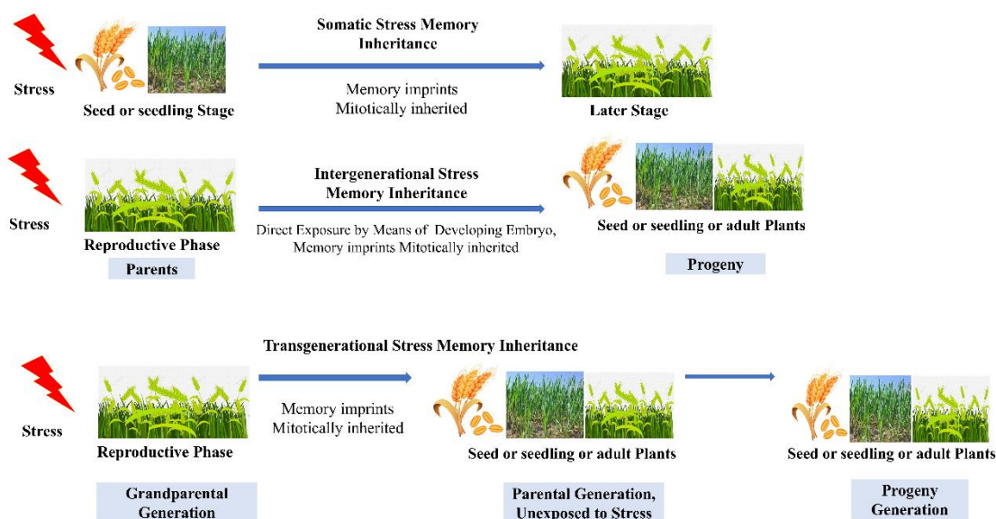
شکل ۳- نحوه توارث انواع حافظه تنش شامل حافظه تنش سوماتیکی، بین نسلی و فرانسلی در گیاهان
