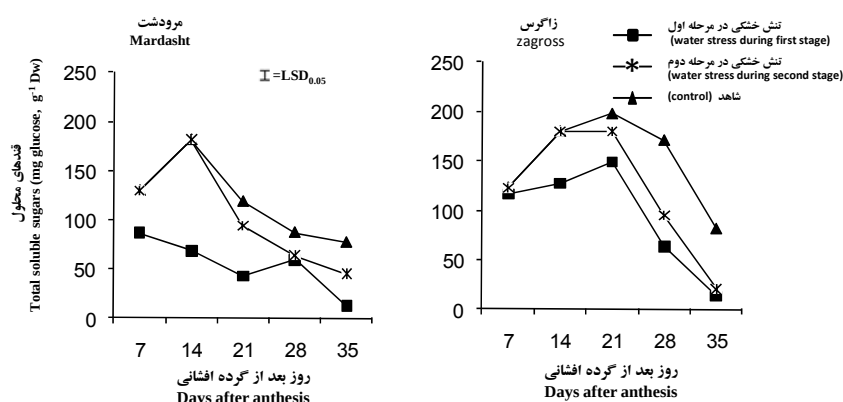
شکل ۳- غلظت قندهای محلول ساقه ارقام گندم زاگرس و مروداشت در مرحله اول تنش خشکی (از شروع گرده افشانی تا ۱۴ روز بعد) و مرحله دوم تنش خشکی (از ۱۴ بعد از گرده افشانی تا زمان برداشت) و شاهد بدون تنش
