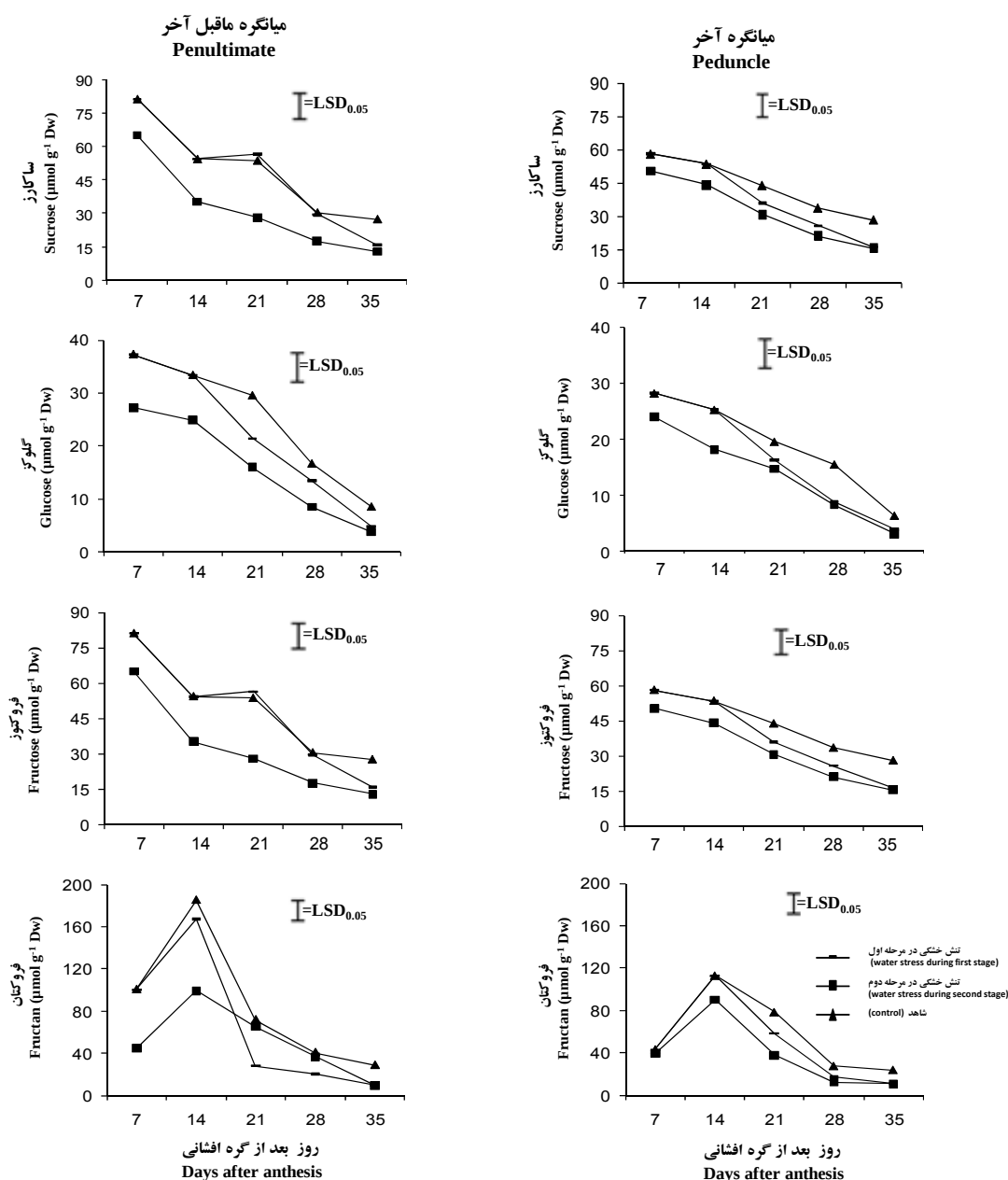
شکل ۵- روند تغییرات غلظت ساکارز، گلوکز، فروکتوز و فروکتان‌های موجود در میانگوه آخر و میانگوه ماقبل آخر در دو رقم گندم زاگرس و مروداشت در تیمار شاهد بدون تنش، تنش خشکی مرحله ۱ (از شروع گرده‌افشانی تا ۱۴ روز بعد) و تنش خشکی مرحله ۲ (از ۱۴ روز بعد از گرده‌افشانی تا پایان دوره رشد گیاه). ا: شاخص تفاوت معنی‌داری LSD در سطح پنج درصد
