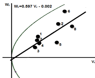
شکل ۳- رگرسیون W_t بر روی V_r برای صفت وزن صد دانه ژنوتیپ‌های برنج
