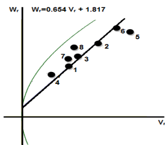
شکل ۶- رگرسیون W_r/V_r روی V_r برای صفت طول خوشه ژنوتیپ‌های برنج (۱: دیلمانی، ۲: طارم محلی، ۳: IR18430-46، ۴: لاین ۲۳، ۵: IR50، ۶: RI18442-1، ۷: RI18447-2، ۸: گیلانه)
