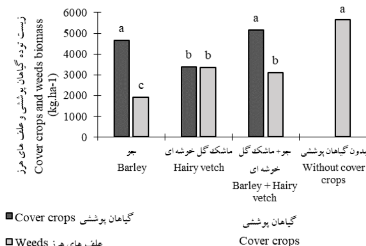
شکل ۱- مقایسه میانگین زیست‌توده گیاهان پوششی و علف‌های هرز در تیمارهای کشت خالص و مخلوط Fig. 1. Mean comparison of biomass of cover crops and weeds in sole and intercropping treatments
